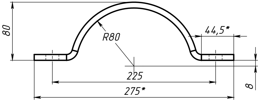
Поз.4 (Полухомут)
