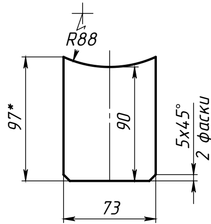
Поз.3 (Ребро среднее)
